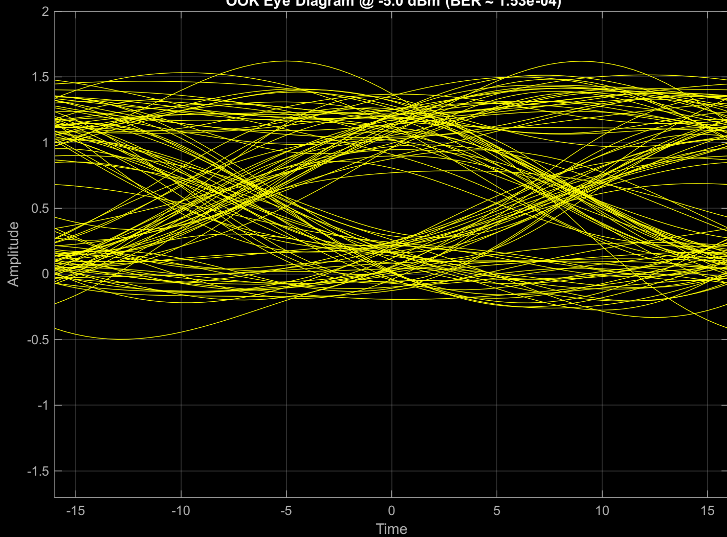
OOK Eye Diagram @ -5.0 dBm (BER \approx 1.53\text{e-}04 )
